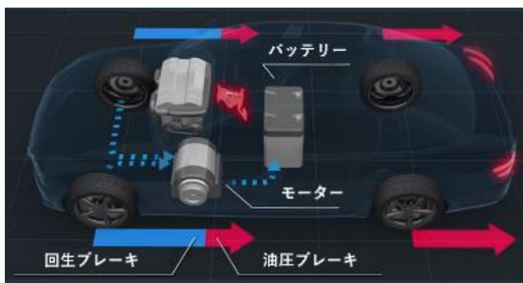
回生協調ブレーキシステム
